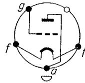
Sockelschaltchema
